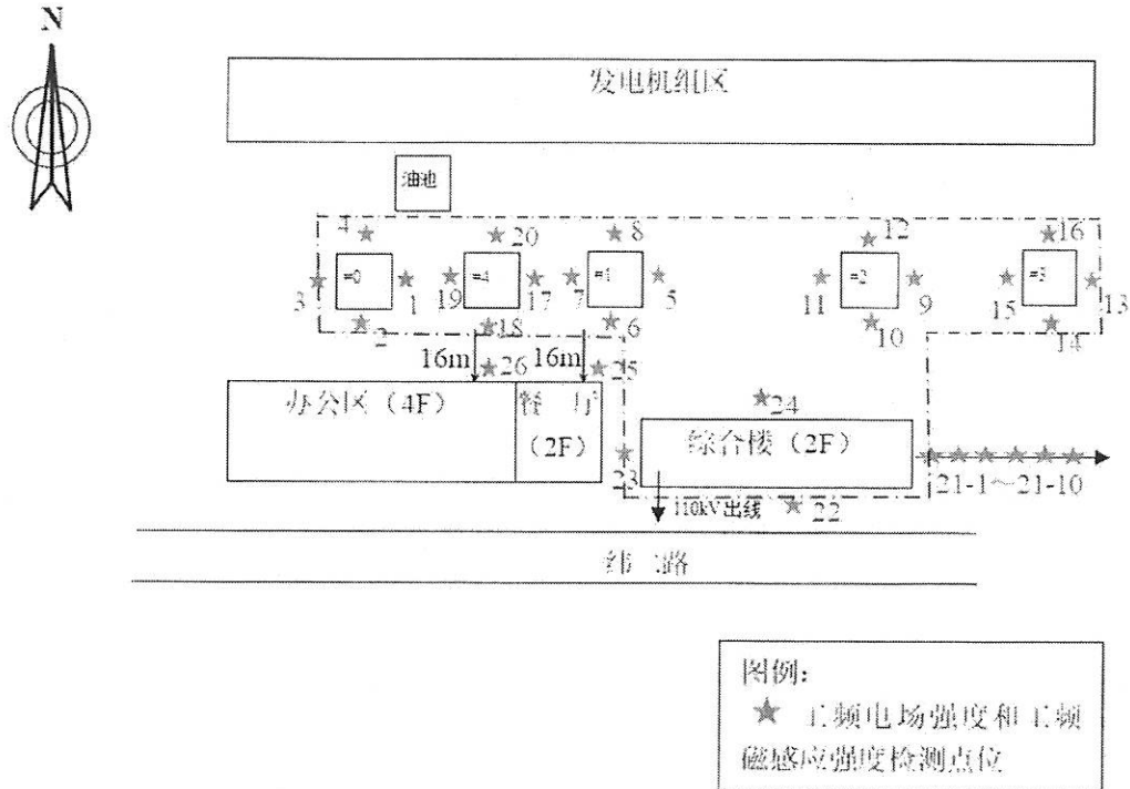
图 1 发电 110kV 升压站检测布点示意图
