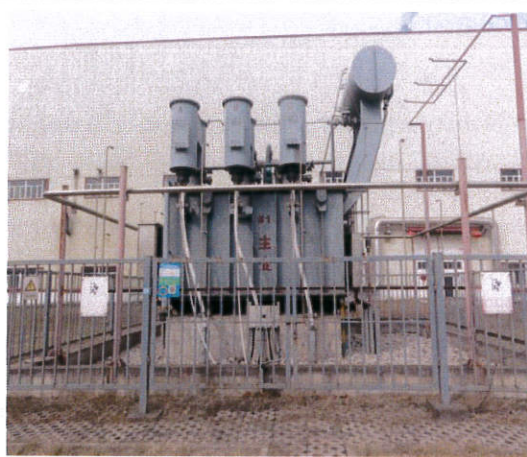
图 4-10 1#主变压器
